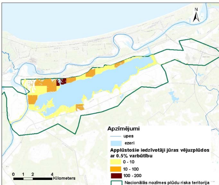
1. attēls. Iedzīvotāju blīvums applūstošajā Babītes ezera polderu teritorijā jūras vējuzplūdos ar varbūtību: 10% (augšā) un 0.5% (lejā)
