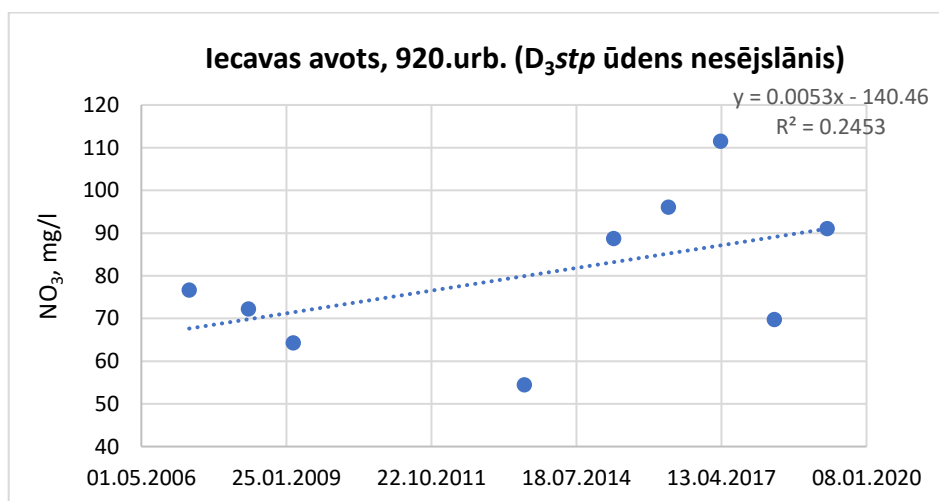
2.attēls. Nitrātjonu koncentrācijas izmaiņas novērojumu punktā Iecavas avota laika posmā no 2006.gada līdz 2020.gadam ar nenozīmīgu augšupejošu tendenci
