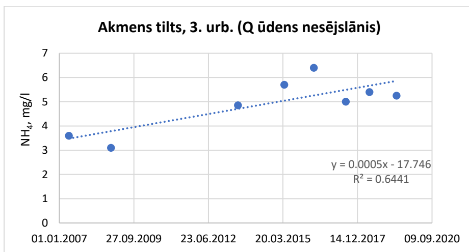
1.attēls. Amonija jonu koncentrācijas izmaiņas novērojuma punktā Akmenis tilts, 3 laika posmā no 2007.gada līdz 2020.gadam ar nozīmīgu augšupejošu tendenci
