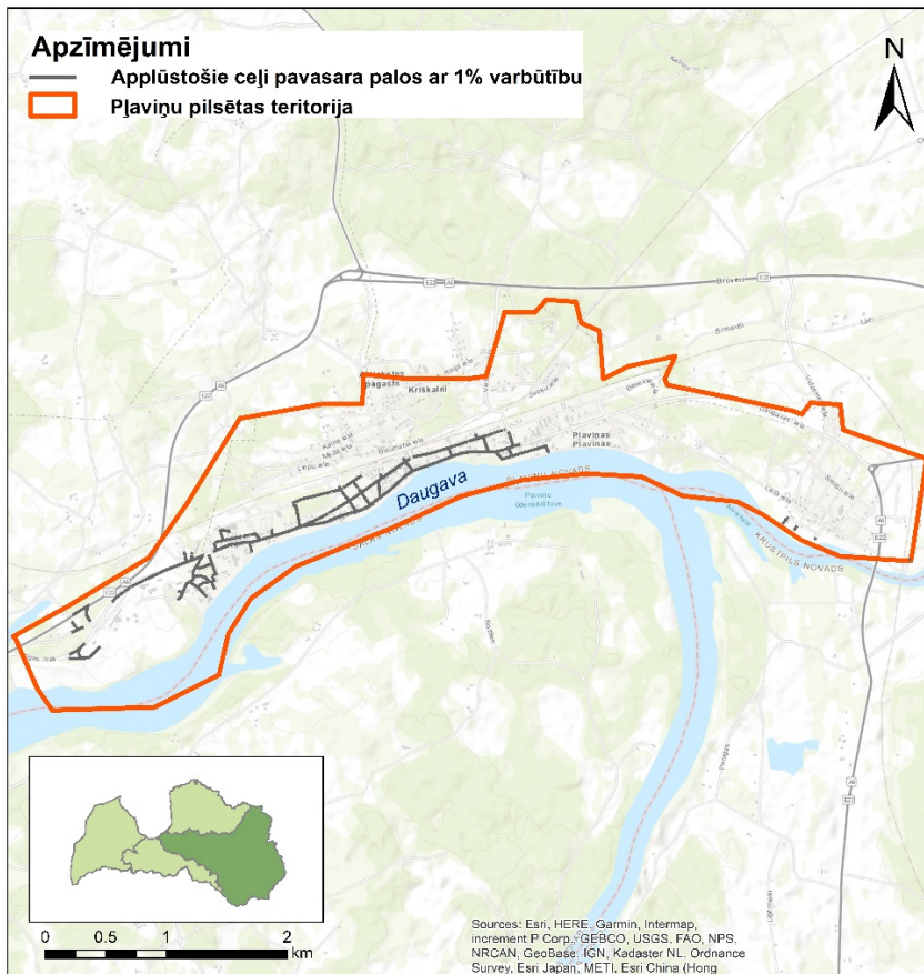
3.attēls. Aplūstošie ceļi Pļaviņu pilsētā pavasara palos ar 1% pārsniegšanas varbūtību
