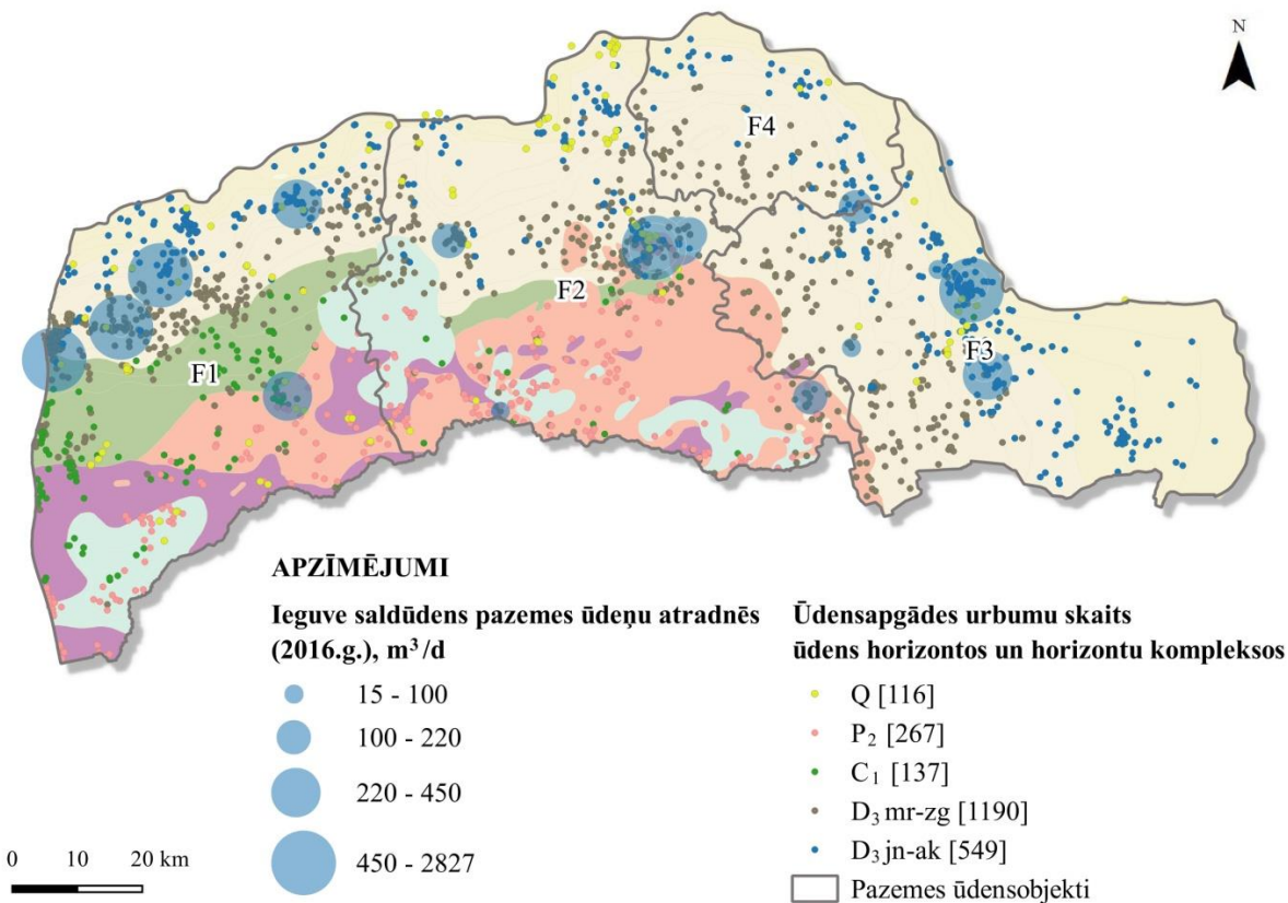
6.attēls. Ūdensapgādes urbumi un saldūdens pazemes ūdeņu atradnēs Famenas ūdens horizontu kompleksa izplatības apgabalā
