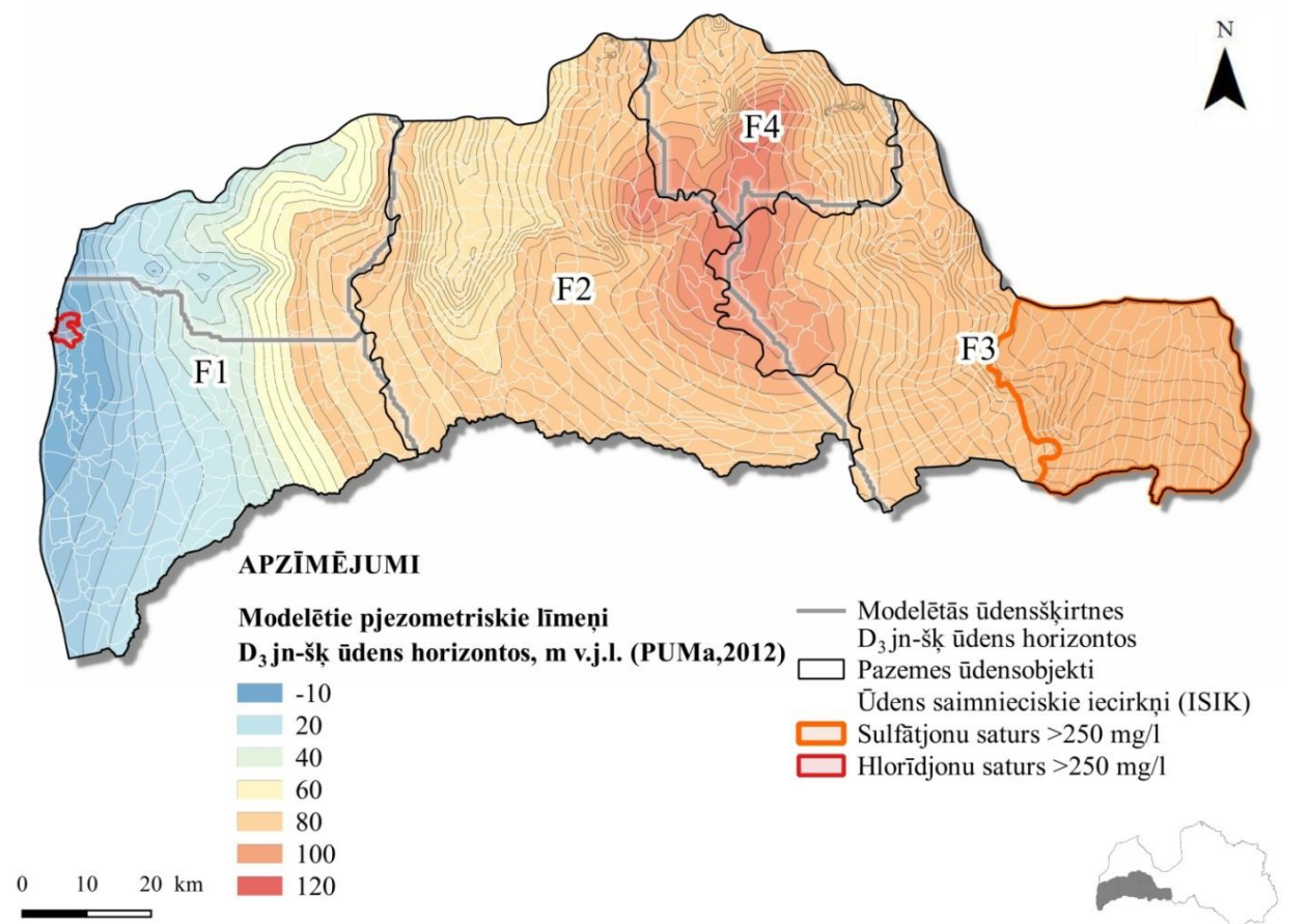
7.attēls. Modelētie pjezometriskie līmeņi Jonišķu-Šķerveļa (D 3 jn-šķ) ūdens horizontu kompleksā Famenas ūdens horizontu kompleksa izplatības areālā
