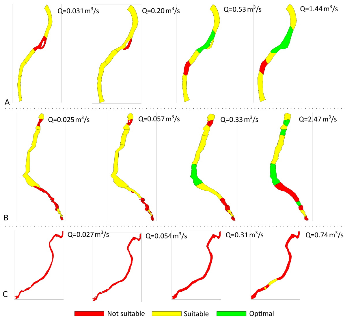
8b. attēls. Sapalam Squalius cephalus pieejamā biotopu platība pie dažādiem caurplūdumiem Bērze – Bikstu-Palejas HES (A), Īsīce – Rundāles HES (B), Auce – Bēne HES (C)
