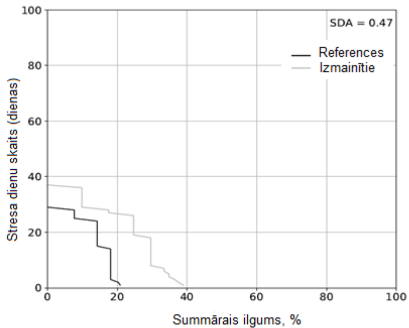
10. attēls. Pieauguša baltā sapala ( Leuciscus leuciscus ) summārais “stresa dienu” ilgums references (dabiskos) un izmainītos apstākļos Īslīces upē, lejpus Rundāles HES.
