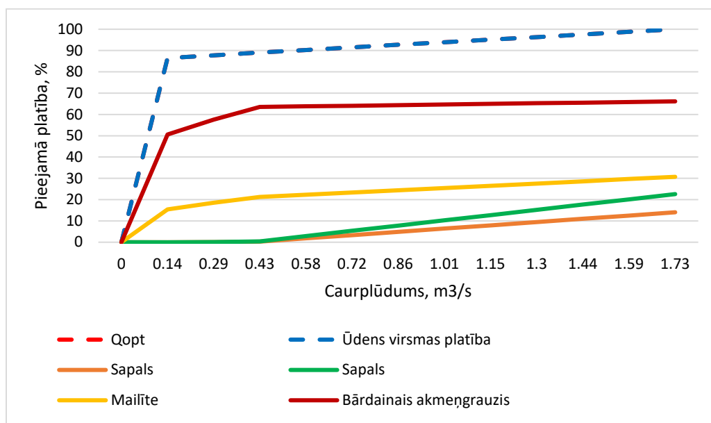
11. attēls. Biotopu un caurplūduma mijiedarbības līkne Aucē, lejpus Bēnes HES
