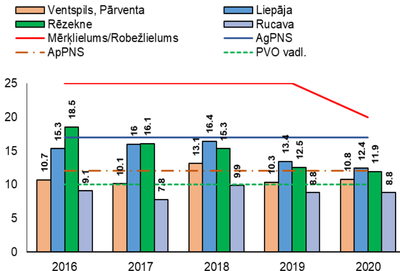
31.attēls. Daļiņu \text{PM}_{2.5} gada vidējās koncentrācijas \mu\text{g}/\text{m}^3 Latvijas pilsētās, 2016.-2020.g.
