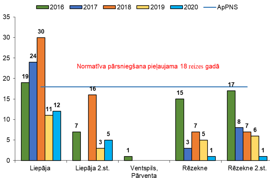
23.attēls. Slāpekļa dioksīda stundas vērtības ApPNS pārsniegšanas gadījumu skaits Latvijas teritorijā, 2016.-2020.g.
