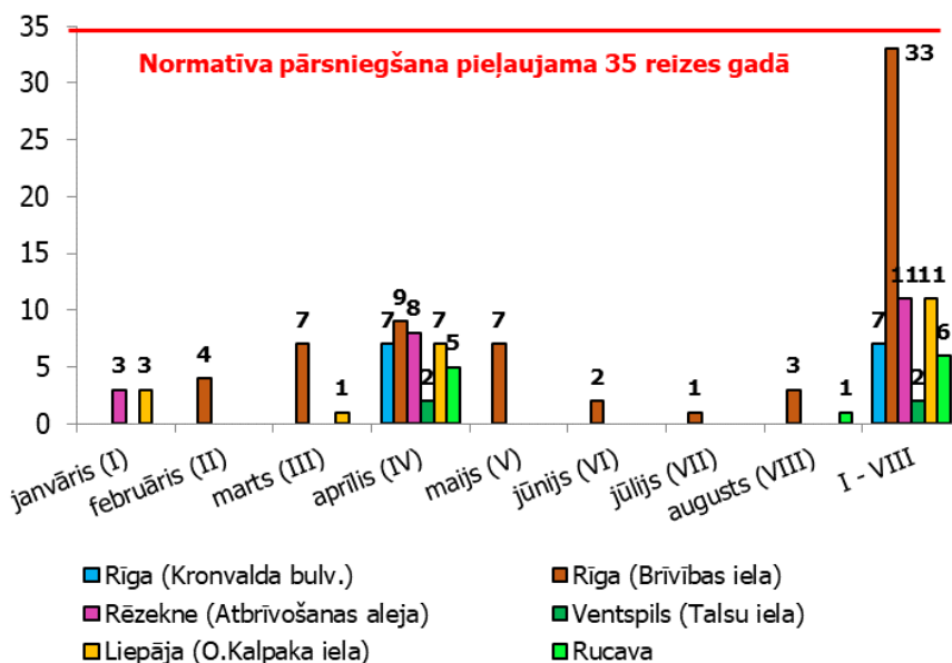
2019.gada daiļiņu PM 10 diennakts normatīva (50 µg/m 3 ) pārsniegšanas gadījumu skaits
